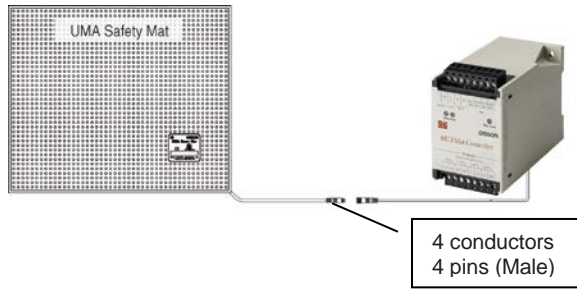
Single 1-Cable Mat (UM□□A-□-□-1)
